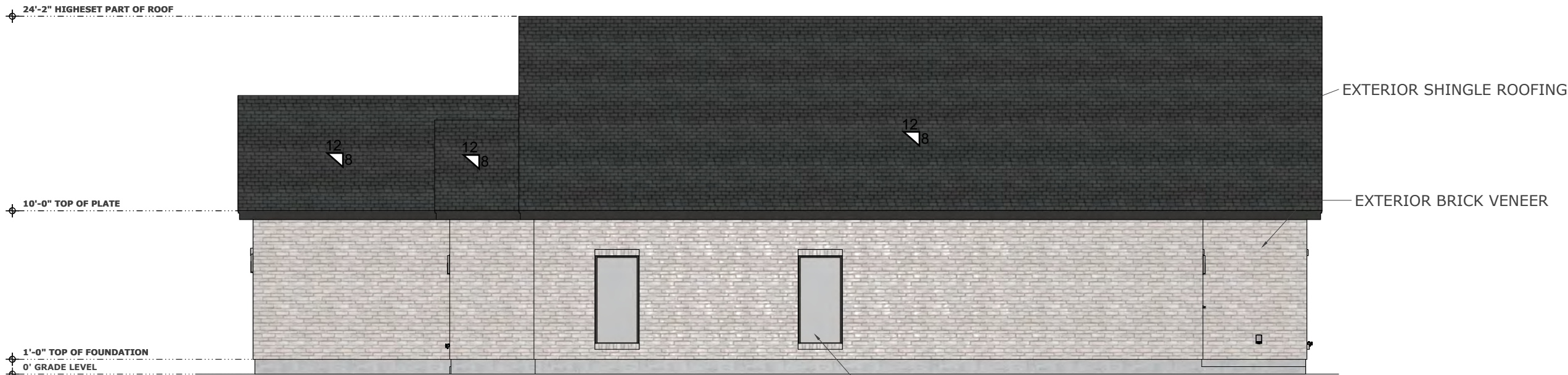
Right Elevation
